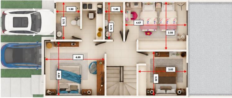
PLANTA ALTA
